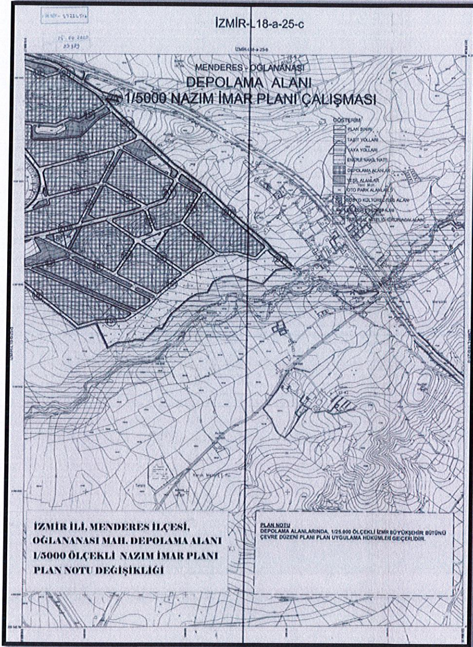
Şekil 8: 1/5.000 Ölçekli Nazım İmar Planı
